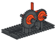
Kurbelgetriebe 2 / Crank gear 2 / Mécanisme à manivelle 2 / Krukasoverbrenging 2 / Mecanismo de manivela 2 / Engrenagem de manivela 2 / Ingranaggio a manovella 2 / Кривошипный механизм 2 / 曲柄传动机构 2 ..... 16
